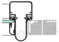
KFI Pfostenprofil
