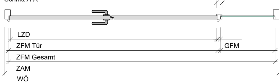
Schnitt A-A
