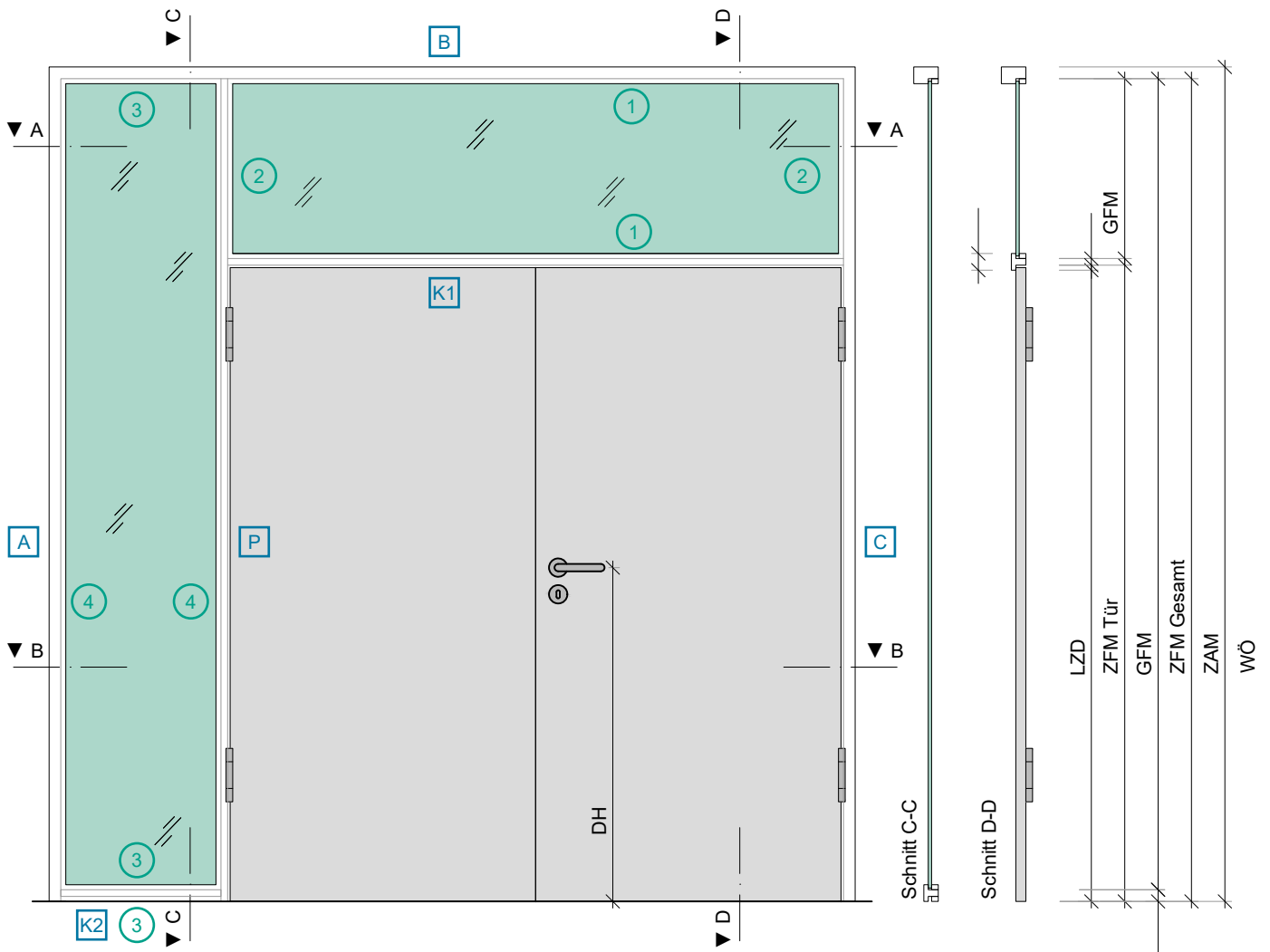
Schnitt A-A
