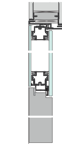
Vertikalschnitt Oberlichtblende GVF70-B
