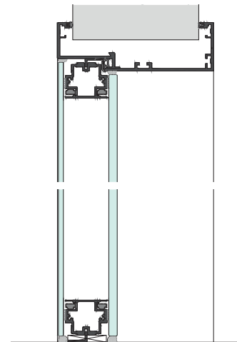
Vertikalschnitt Seitenteil GVF70-S
