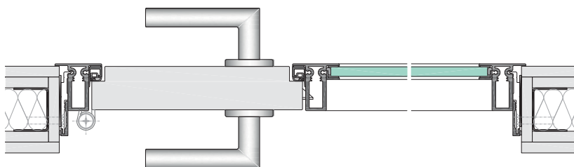
1-flg. Türblatt mit Glasseitenteil in Blockzarge TLS39-A8 mit partieller Leibungsverklebung
