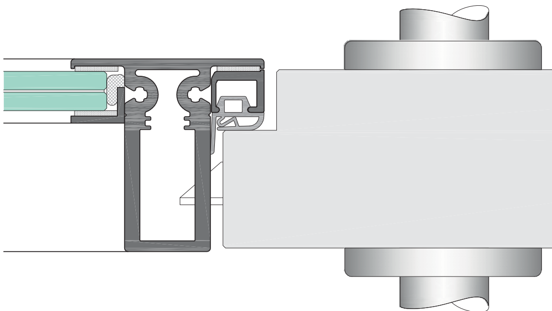
Türblatt mit Aluminiumzarge TLS als Pfosten / Kämpfer Abmessungen M1:1
