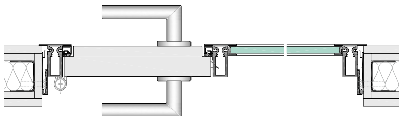
1-flg. Türblatt mit Glasseitenteil in Blockzarge TLS39-A8 mit partieller Leibungsverkleidung
