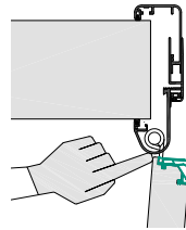
Abgesicherte Scherstellen
