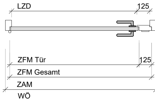
Schnitt A-A
