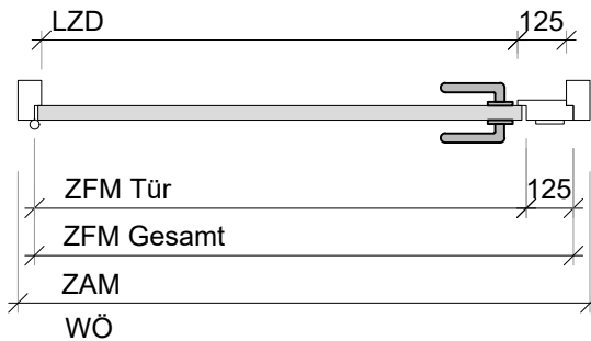
Schnitt B-B
