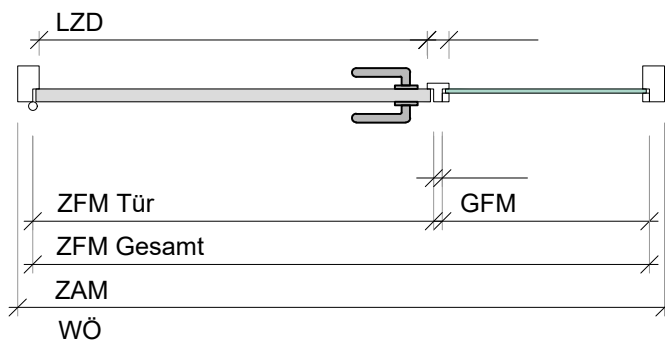
Schnitt A-A
