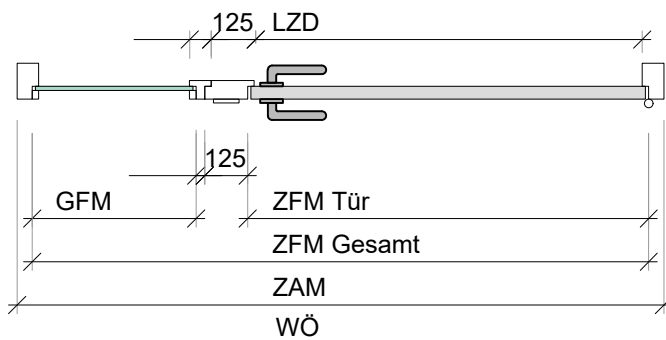
Schnitt A-A
