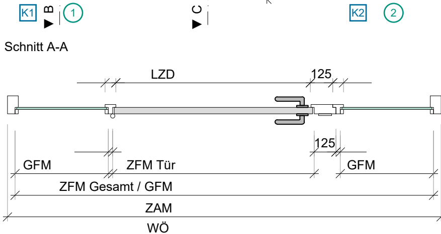
Systemskizze - ohne Maßstab und Details
