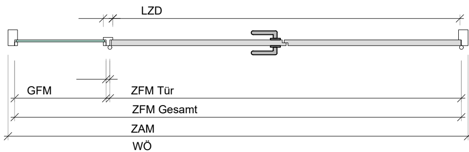
Schnitt A-A
