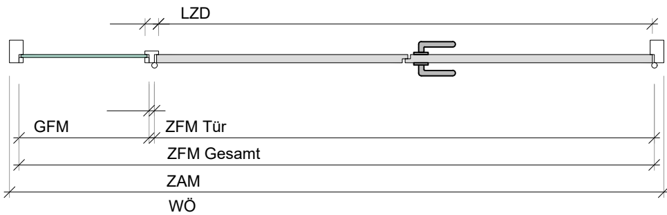
Schnitt A-A
