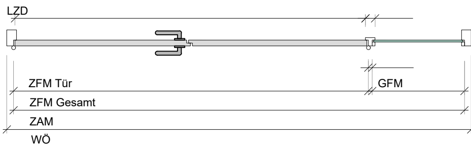
Schnitt A-A
