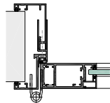
Umfassungszarge Typ EUROKS48
