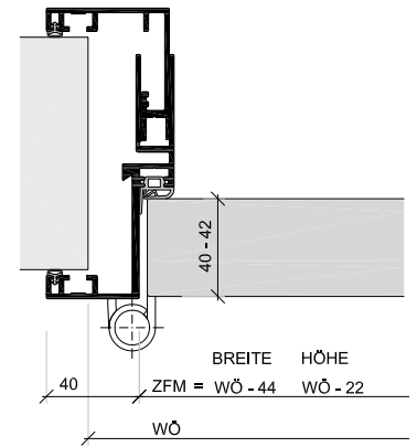
EUROKS48 für stumpfes Türblatt, 40/42 mm
