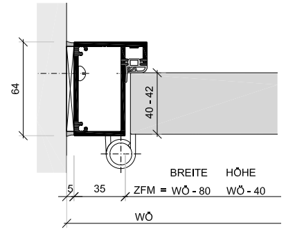
BS48 für stumpfes Türblatt, 40/42 mm
