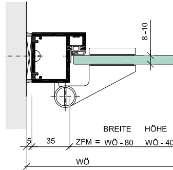
BF30 für Ganzglastür, 8 oder 10 mm
