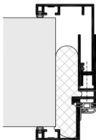
Einbau mit Montageschaum (bauseits) bis Türgewicht 60kg
