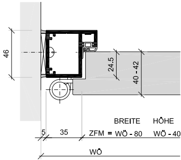
BF30 für gefälztes Türblatt, 40/42 mm (Normfalz)
