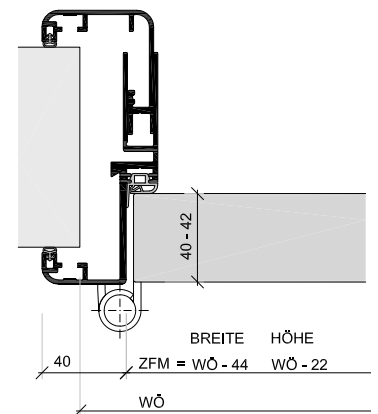
EURORS48 für stumpfes Türblatt, 40/42 mm
