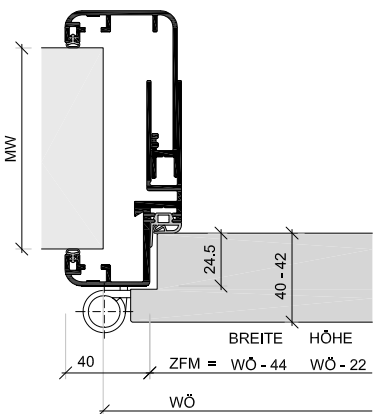
EURORF30 für gefälztes Türblatt, 40/42 mm (Normfalz)
