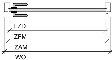
Schnitt A-A
