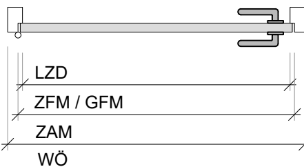
Schnitt B-B
