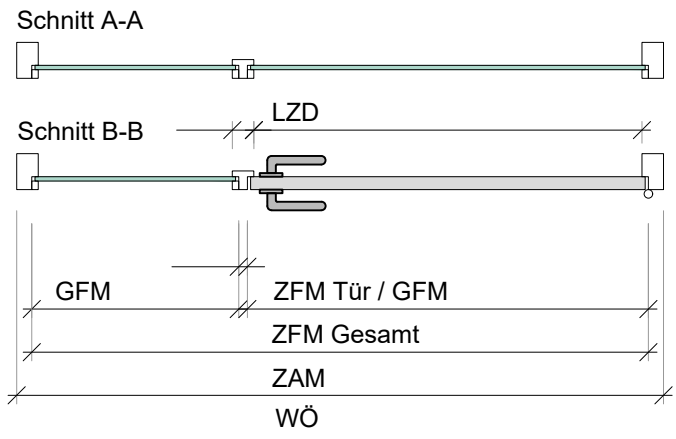
Systemskizze - ohne Maßstab und Details
