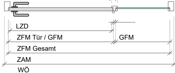
Schnitt B-B
