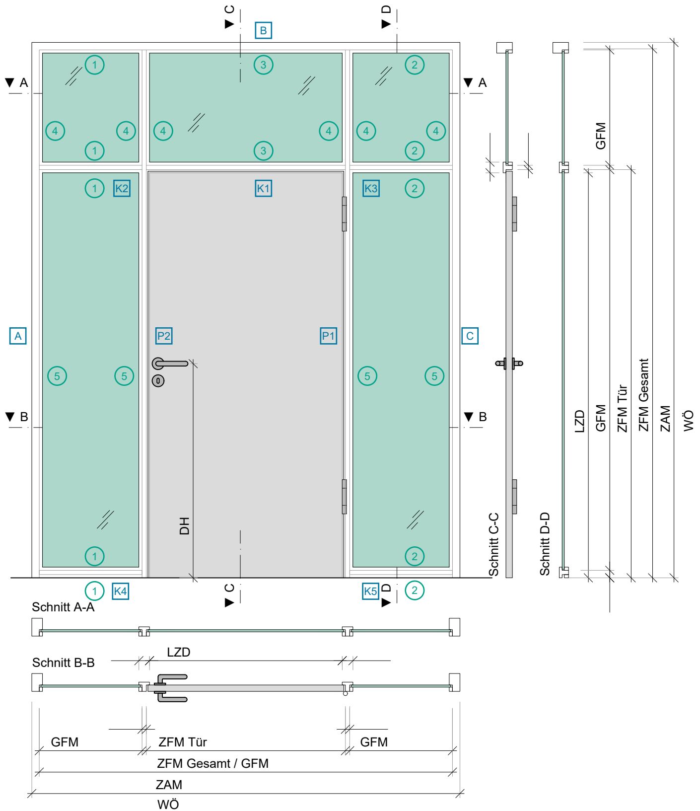
Systemskizze - ohne Maßstab und Details
