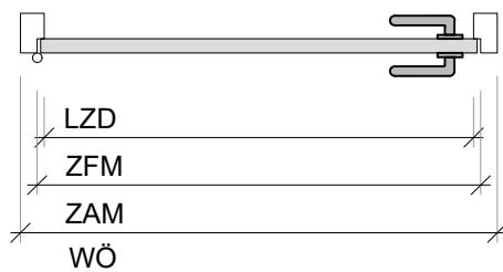
Schnitt A-A
