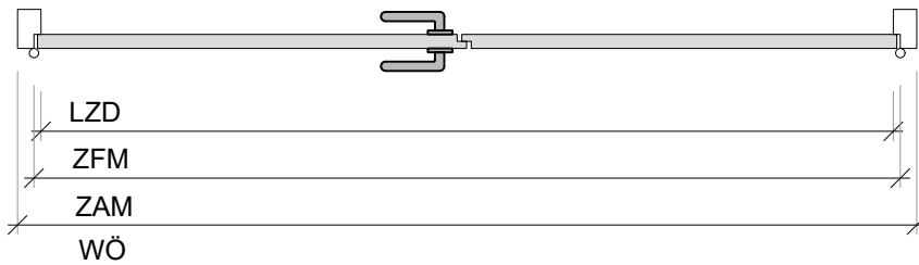
Schnitt A-A
