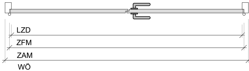
Schnitt A-A
