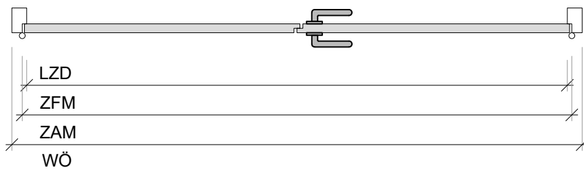
Schnitt A-A
