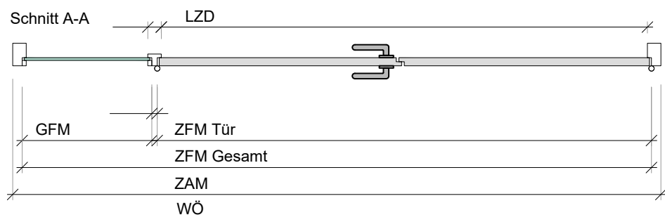
Systemskizze - ohne Maßstab und Details
