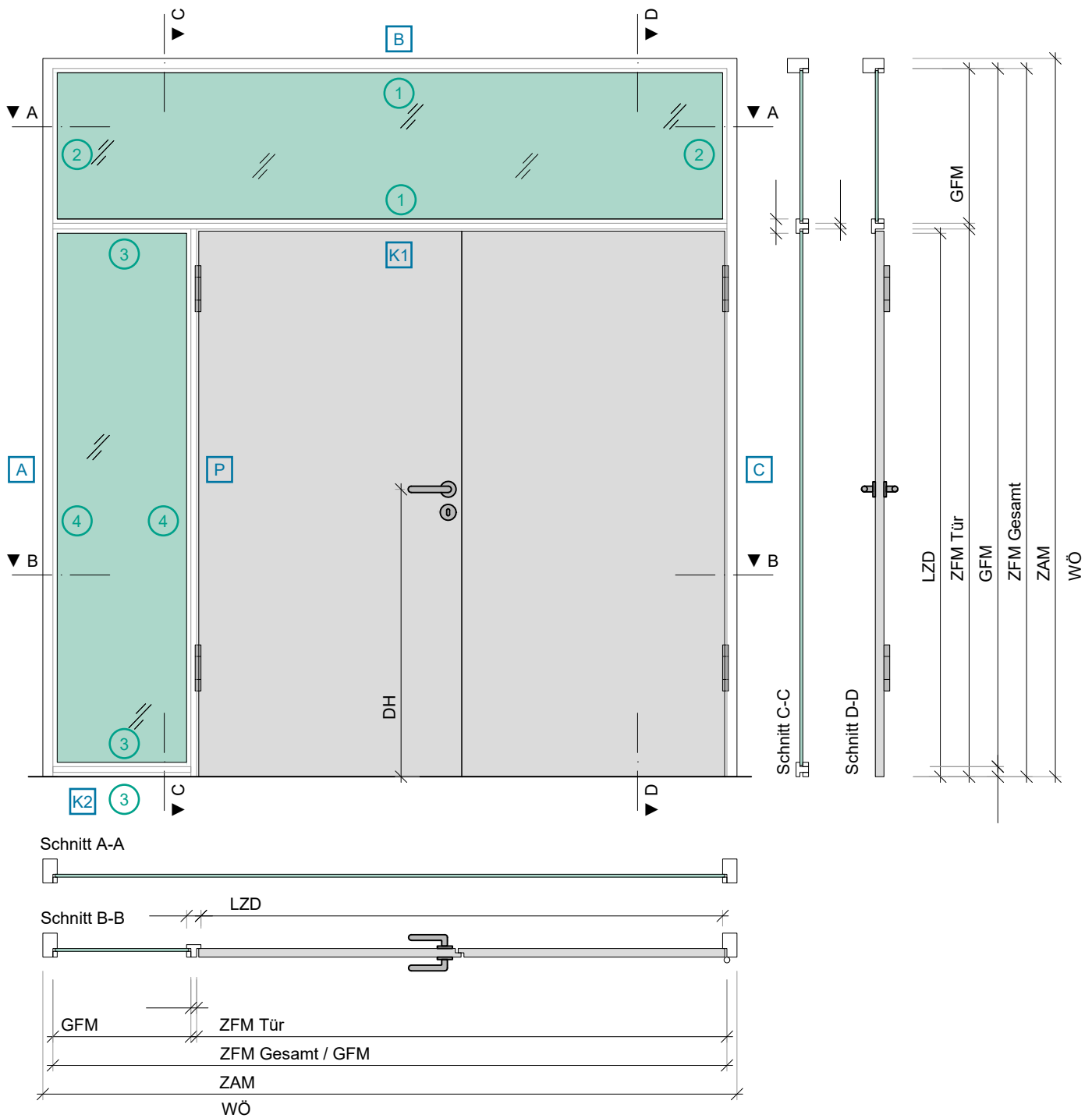
Systemskizze - ohne Maßstab und Details
