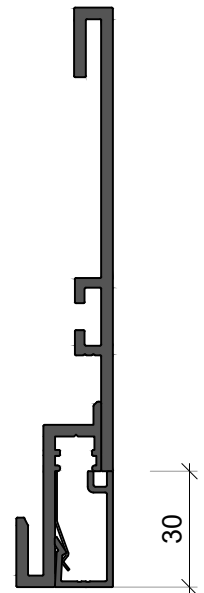
FZS-V Schiebetür / Sliding Door
