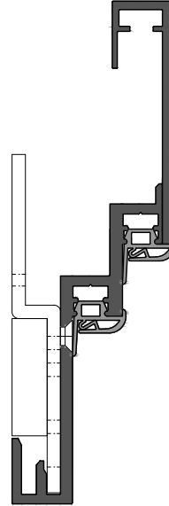
LZDS mit Küffner CP - Band with Küffner CP - Hinge
