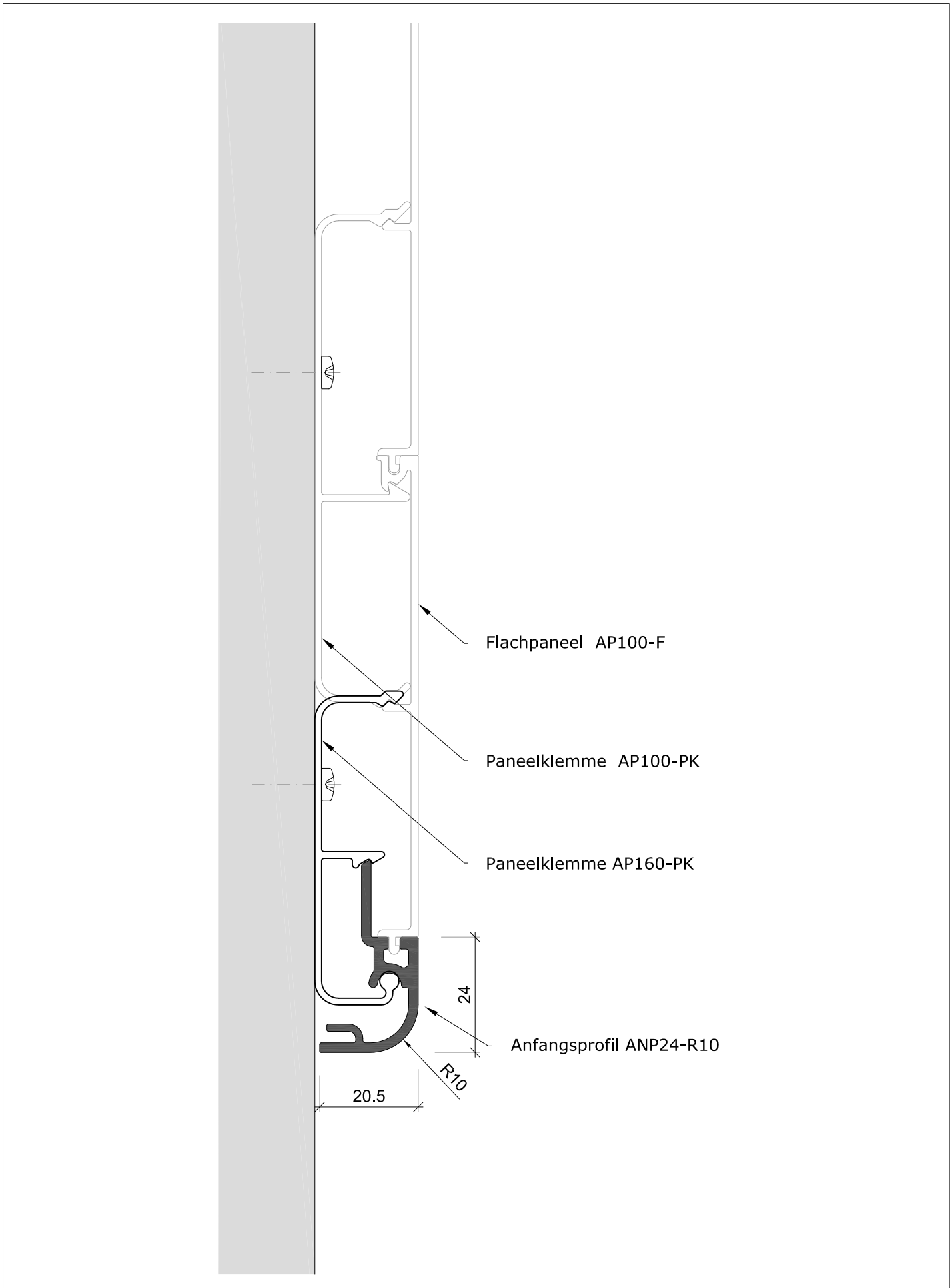
Typ ANP24-R10
