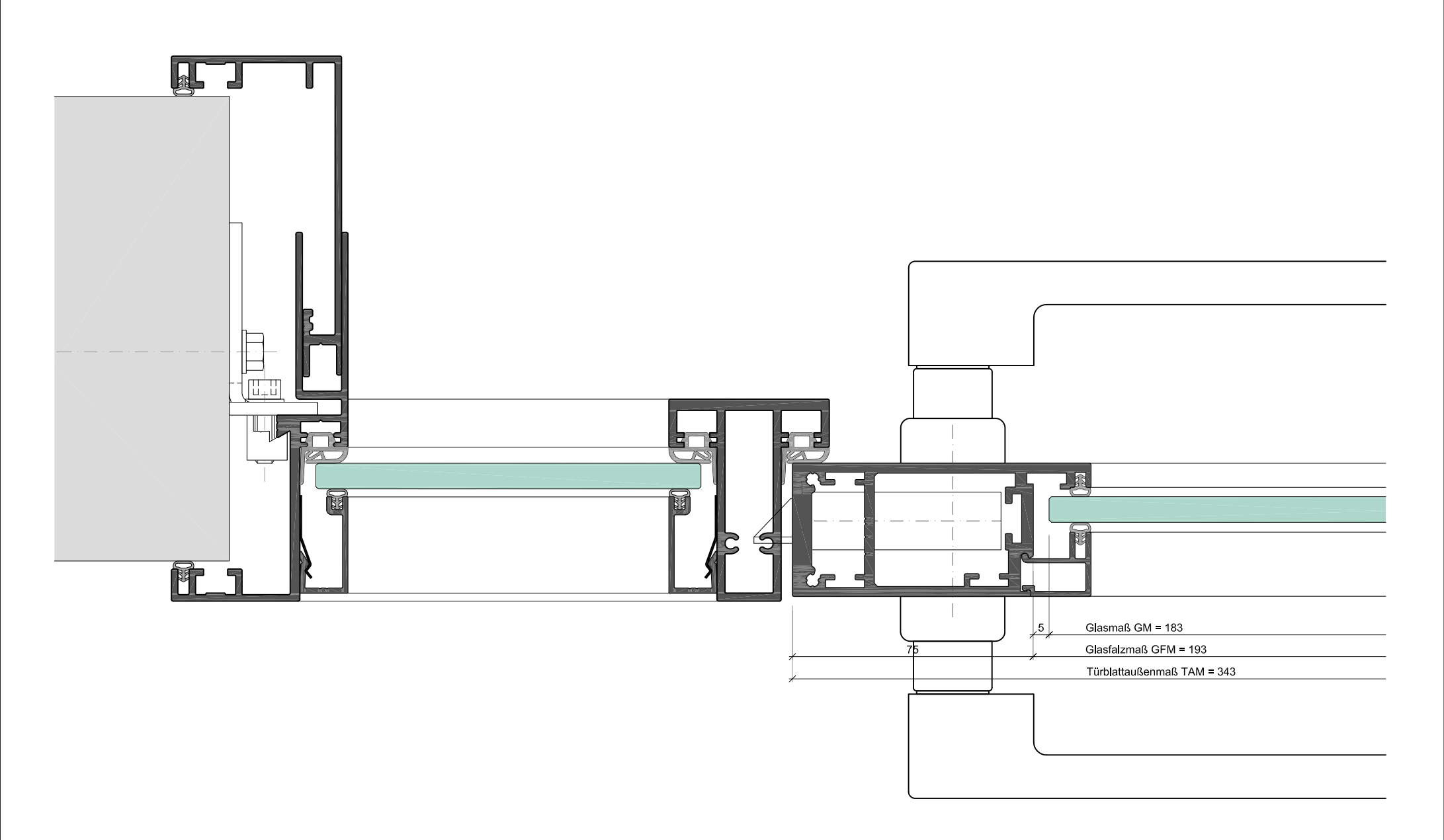
Typ ART42-1-EUROKS-Seitenteil
