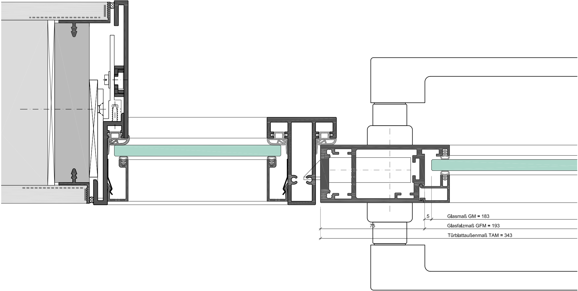
Typ ART42-1-FZS-Seitenteil
