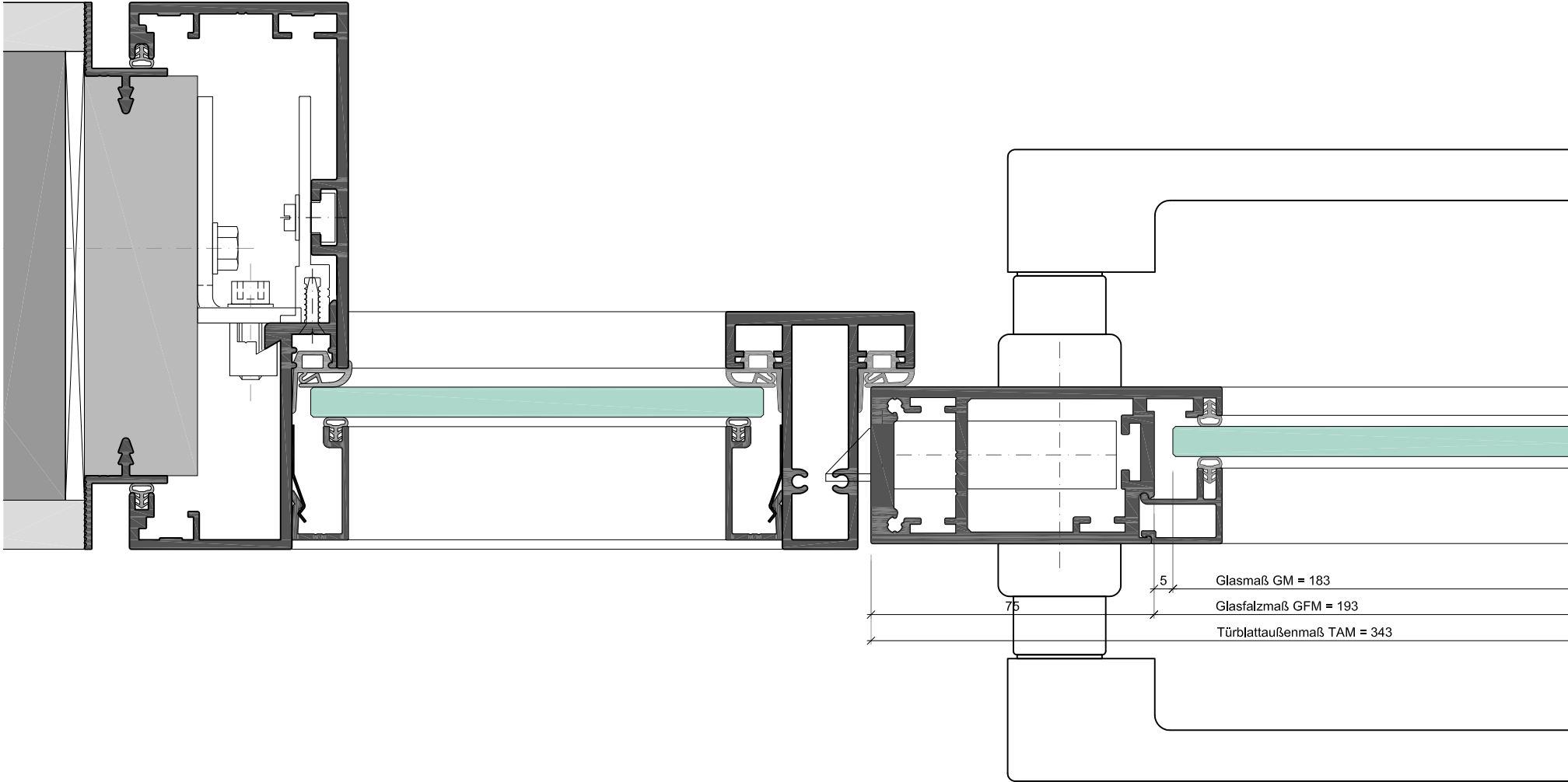
Typ ART42-1-USBV-G-Seitenteil
