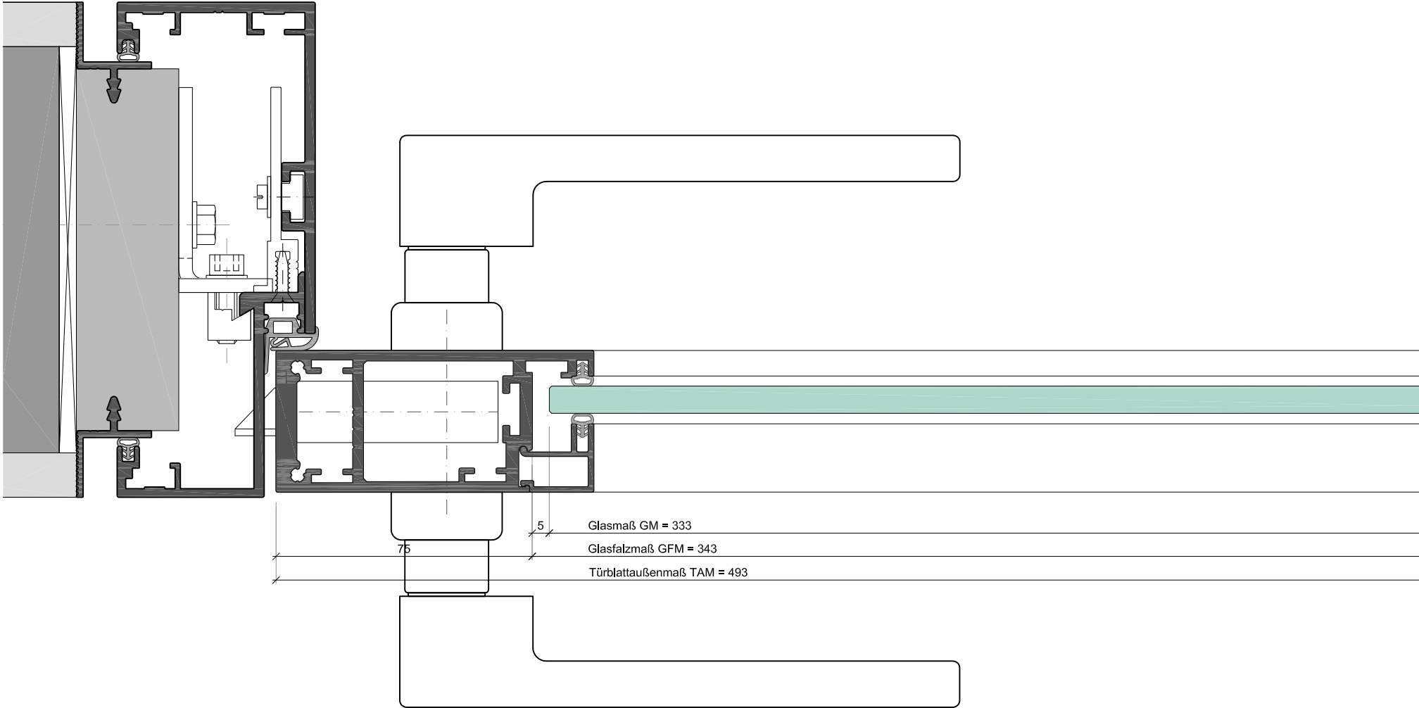
Typ ART42-1-USBV-G
