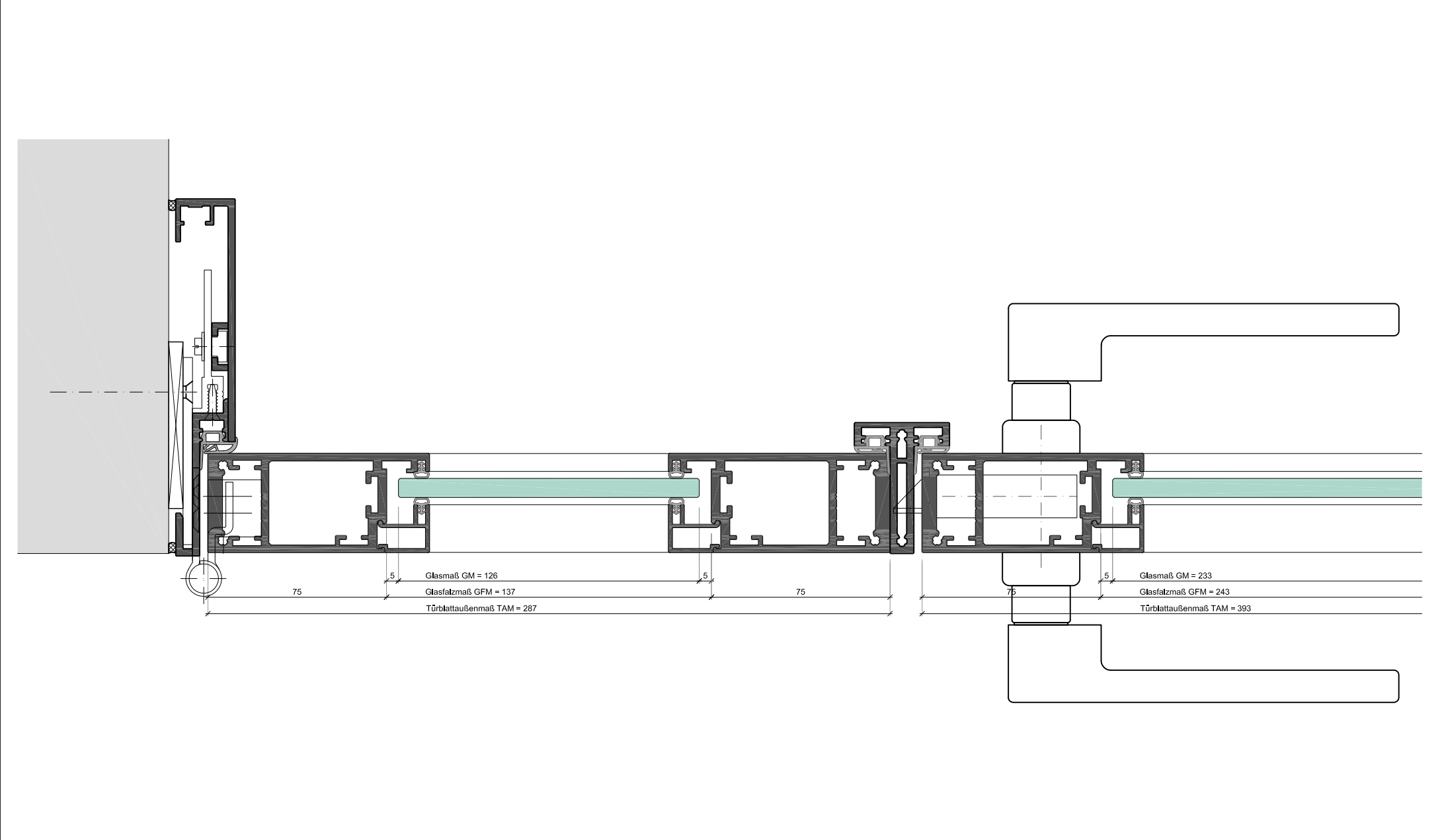
Typ ART42-2-FZSB
