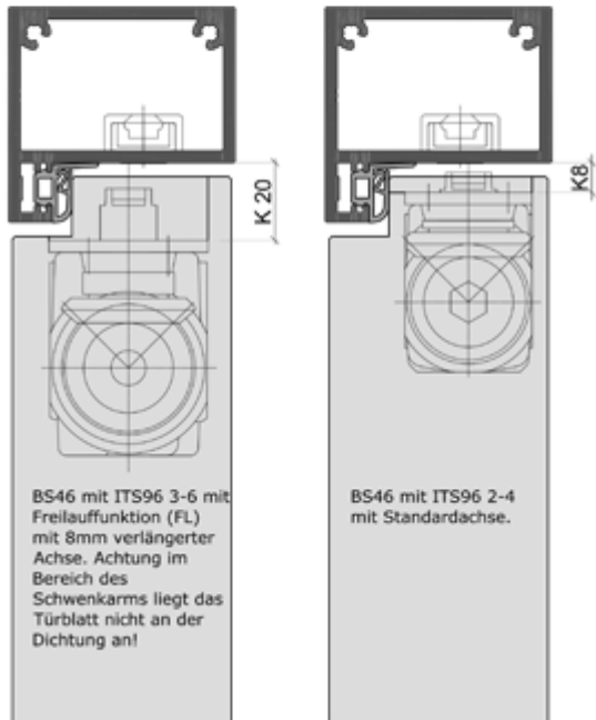
verdeckt liegender Türschließer Dorma ITS 96
