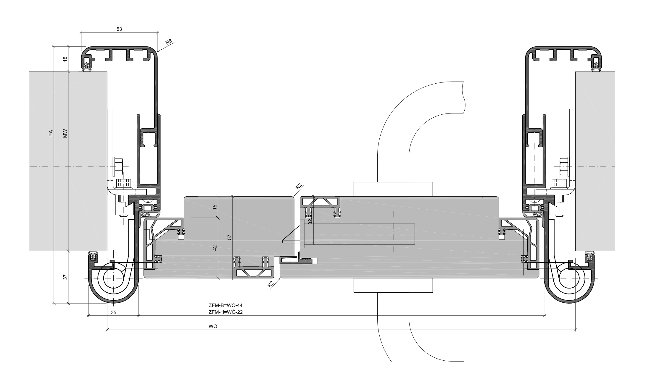
EUROFI48-5-57SL-2FLG
